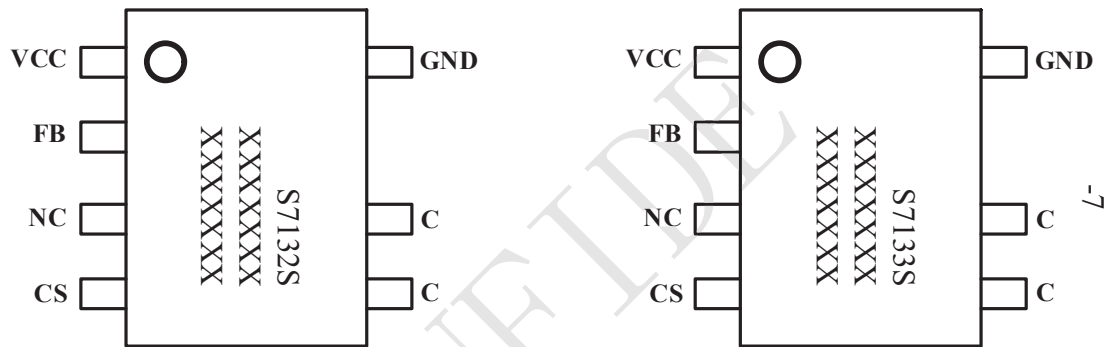
封装管脚图
